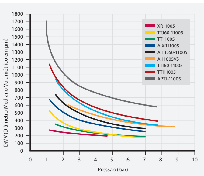
Figura 3. Diâmetros volumétricos de gotas das pontas de pulverização XR, TT, TTJ60, AIXR, AI, AITTJ60, TT160, TTI e APTJ em relação à pressão.
